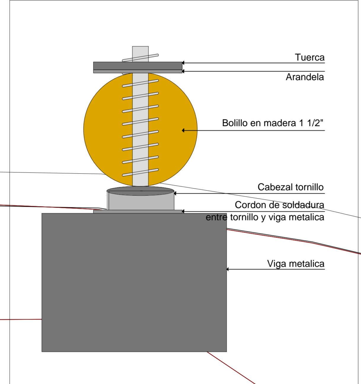
DETALLE FIJACION DE BOLILLO A VIGA METALICA.
