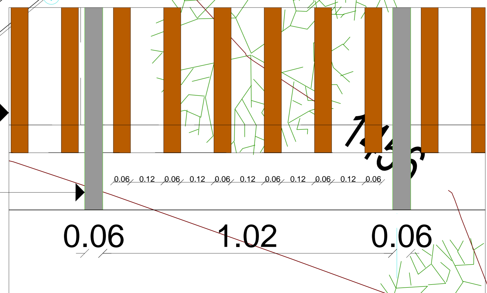
DETALLE LOCALIZACION BOLILLOS.
